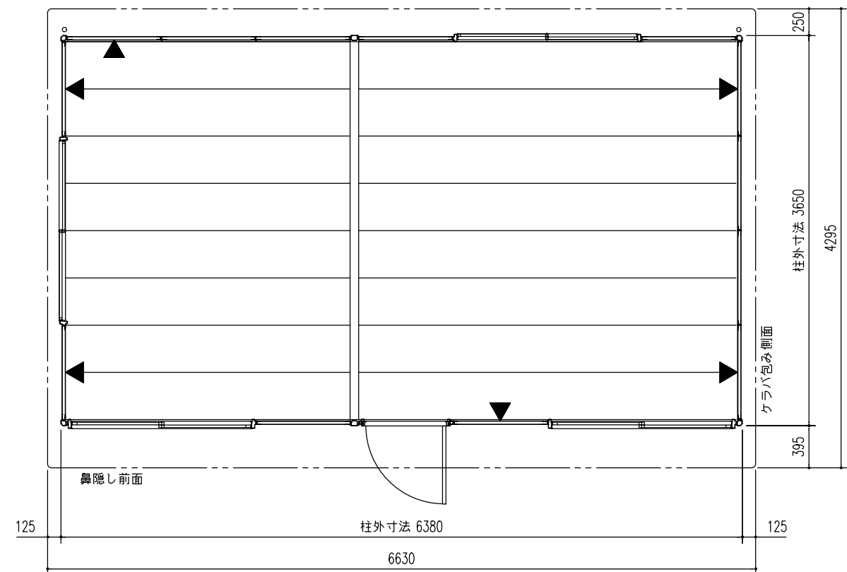
平面図 (S=1/50)
