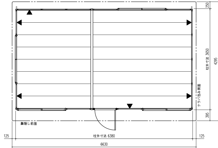
平面図 (S=1/50)
