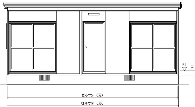
正面立面図 (S=1/50)
