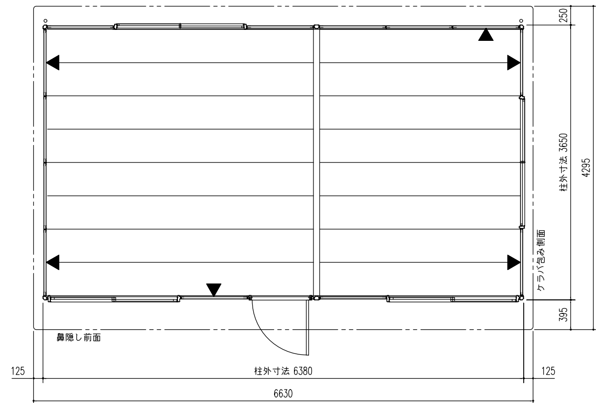
平面図 (S=1/50)
