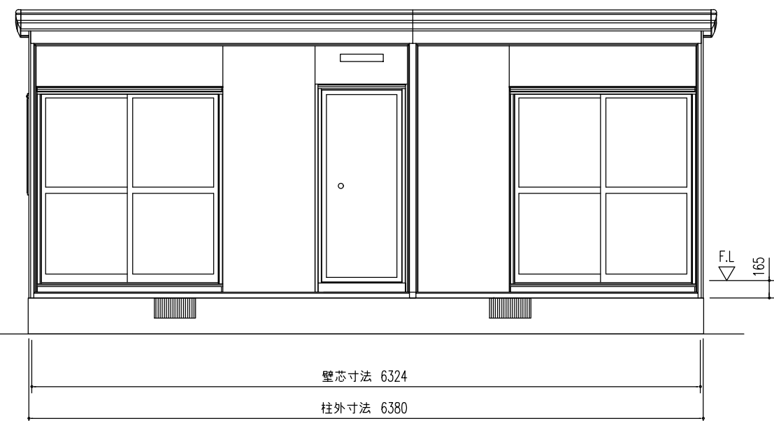
正面立面図 (S=1/50)
