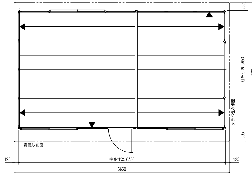
平面図 (S=1/50)
