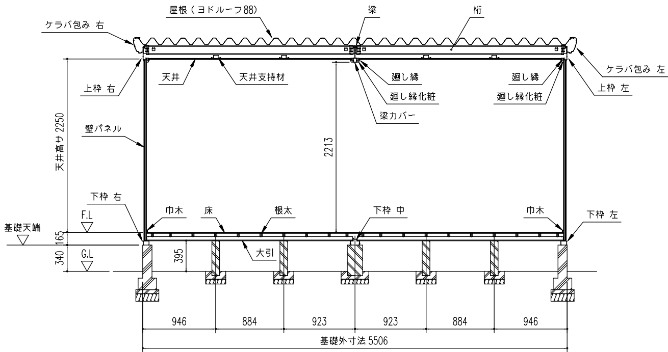
正面断面図 (S=1/50)
