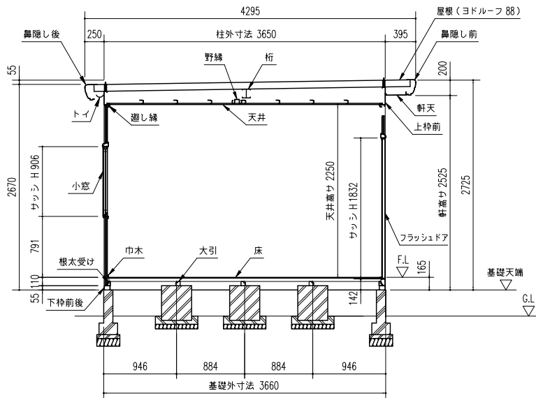
側面断面図 (S=1/50)
