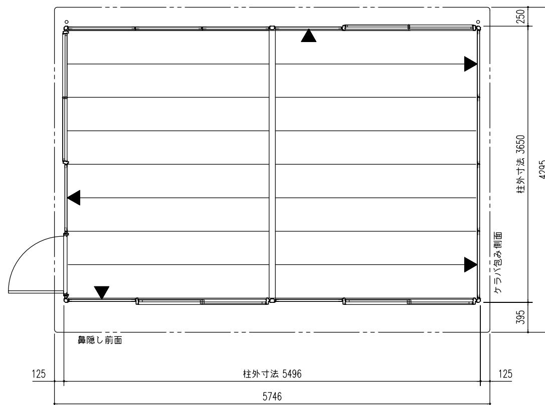
平面図 (S=1/50)
