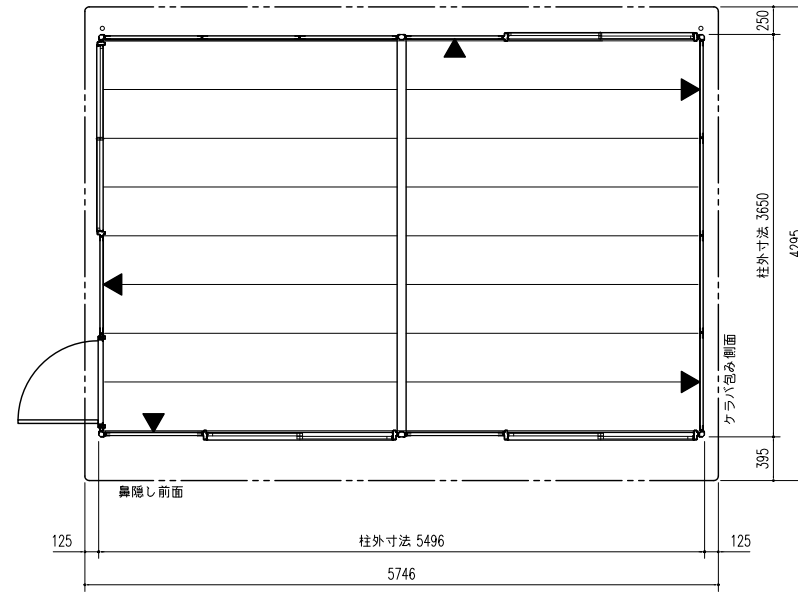
平面図 (S=1/50)
