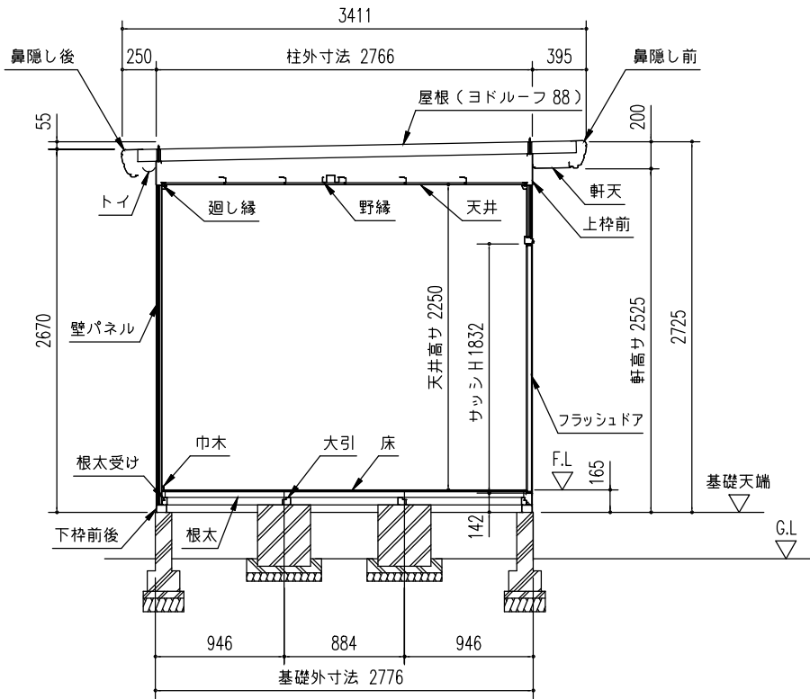
側面断面図 （S=1/50）
