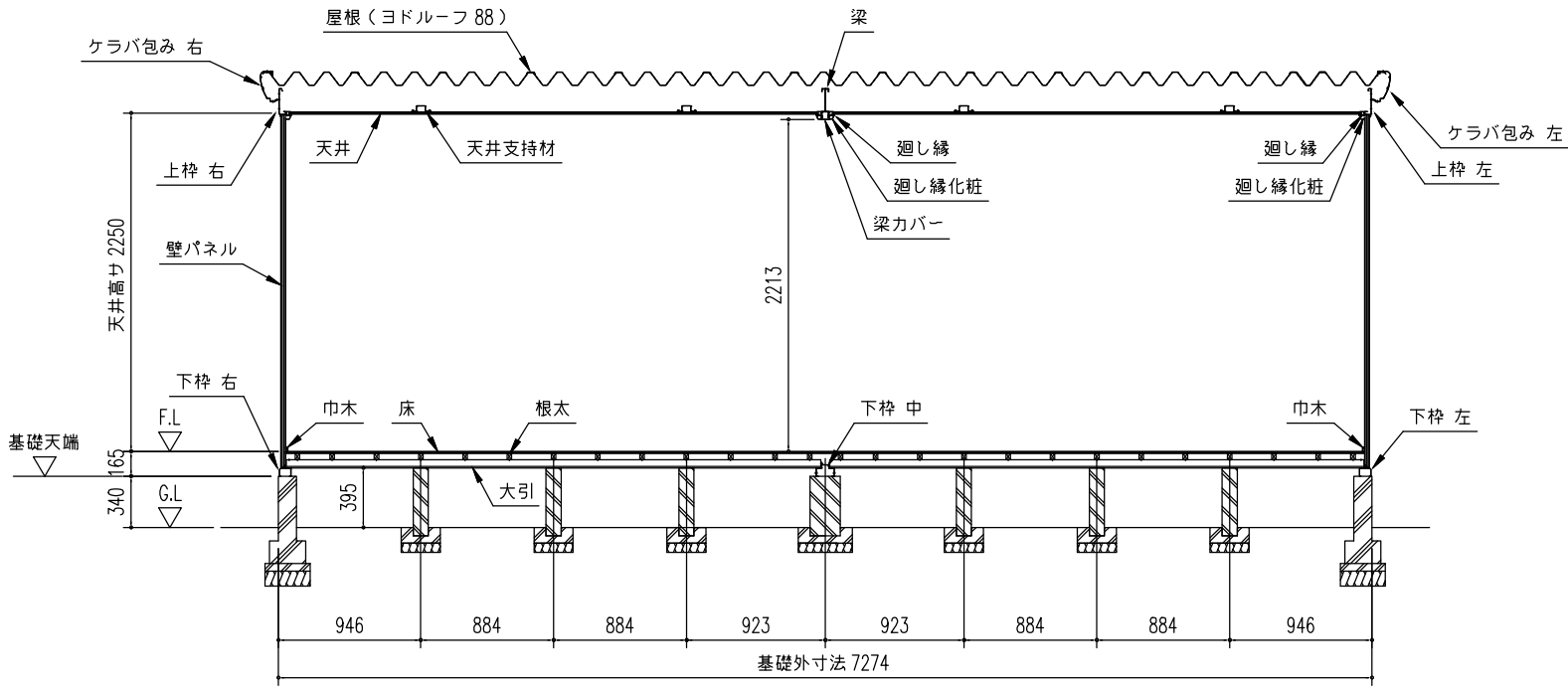
正面断面図 （S=1/50）
