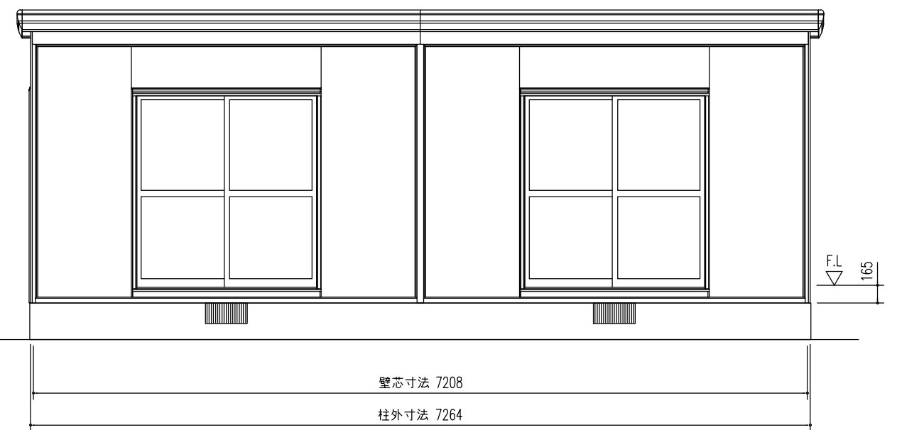
正 面 立 面 図 (S=1/50)
