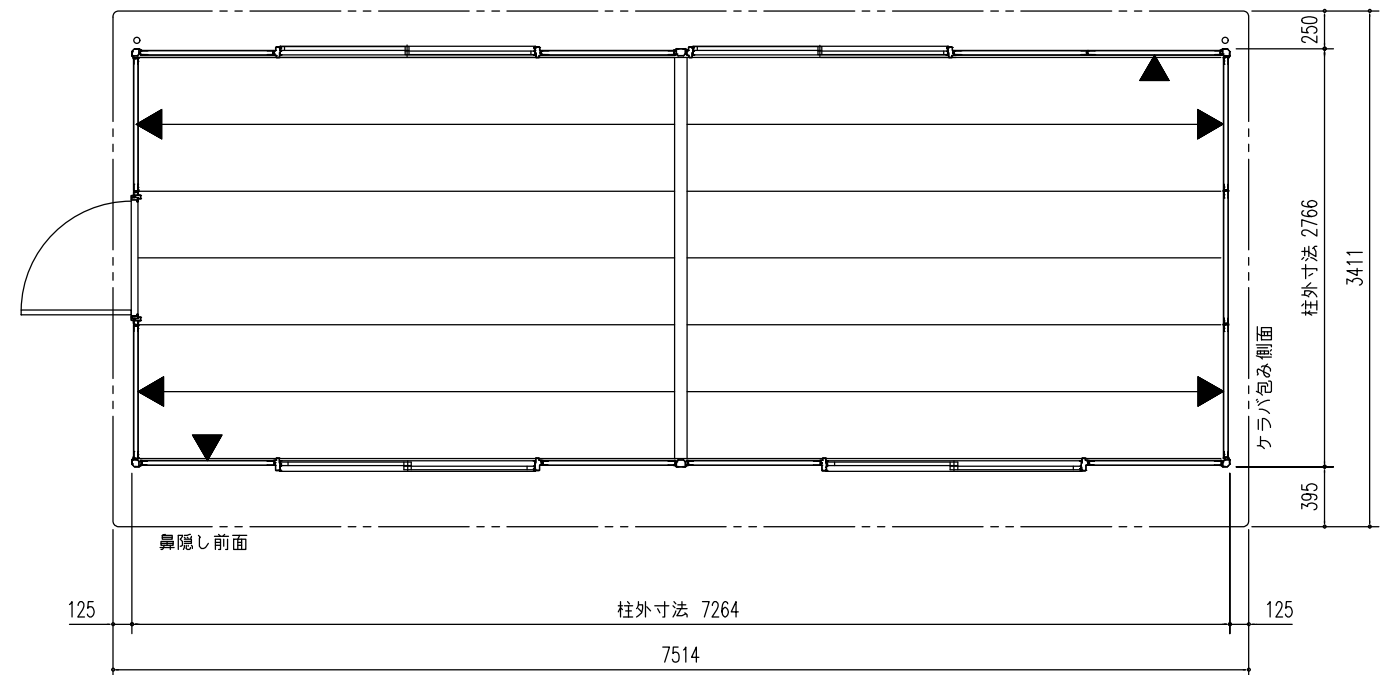
平 面 図 (S=1/50) ▼印はブレースパネルを示す。 間口 2枚 奥行 4枚
