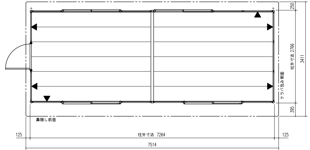
平面図 (S=1/50)
