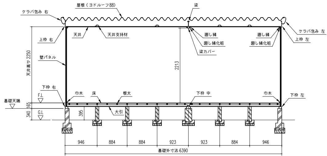
正面断面図 (S=1/50)
