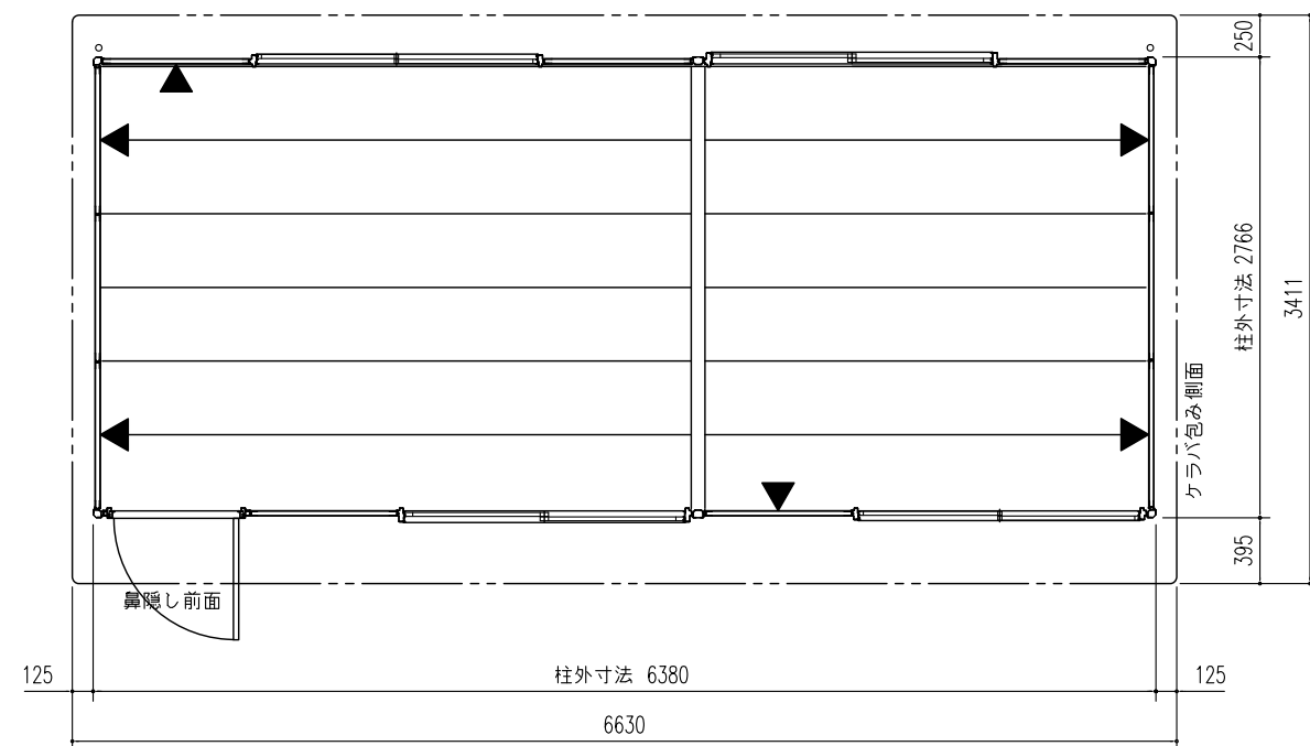
平面図 (S=1/50)
