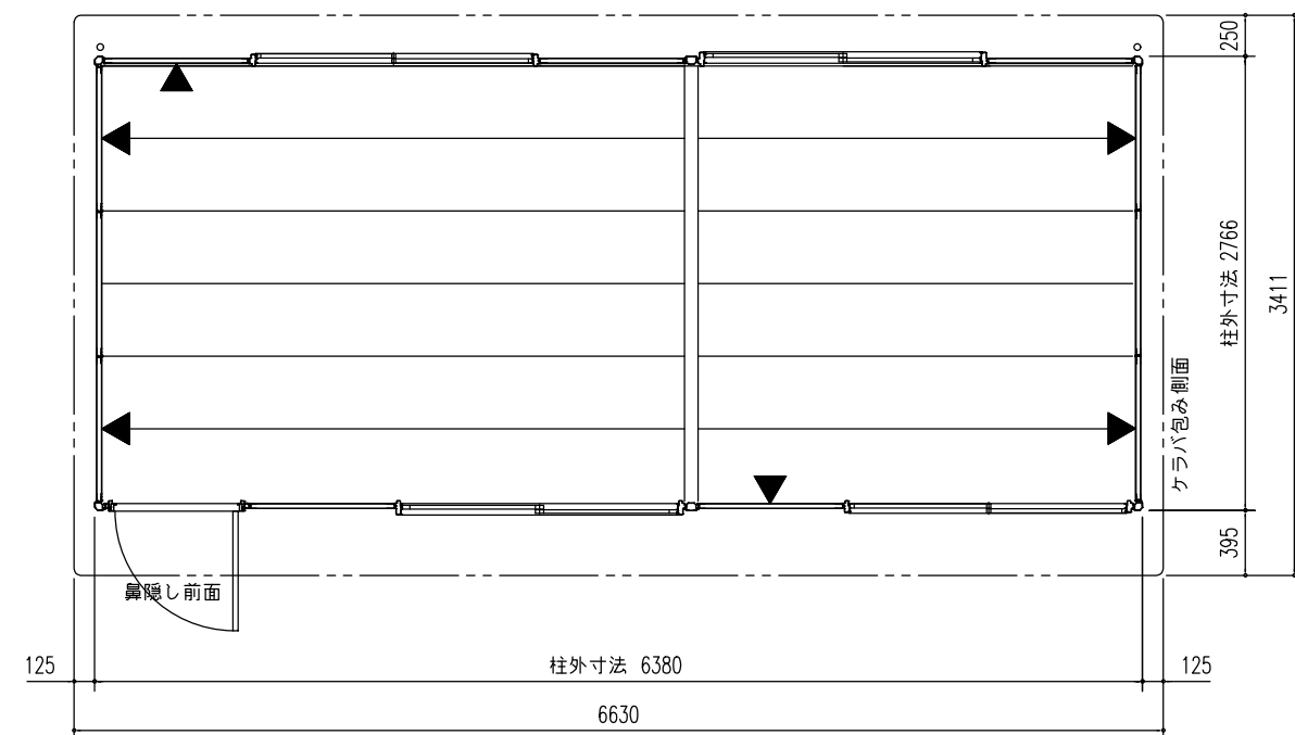
平面図 (S=1/50)
