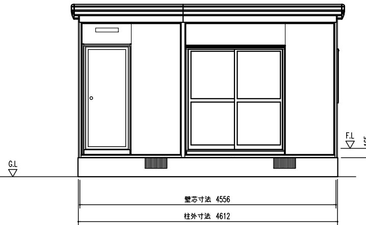
正面立面図 (S=1/50)
