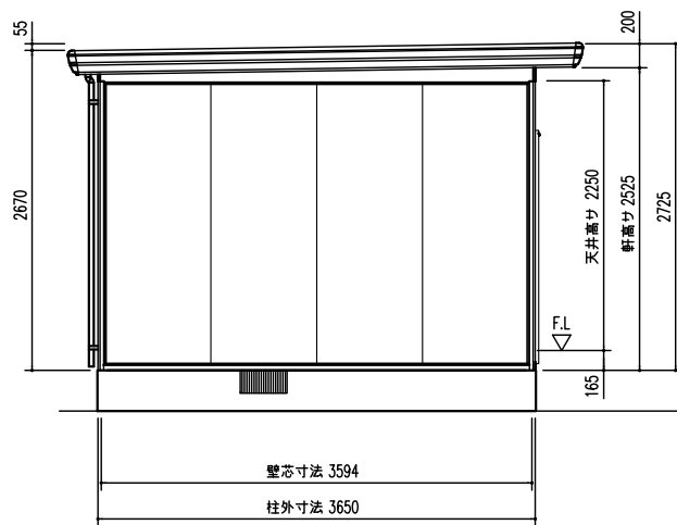
側面立面図 (S=1/50)
