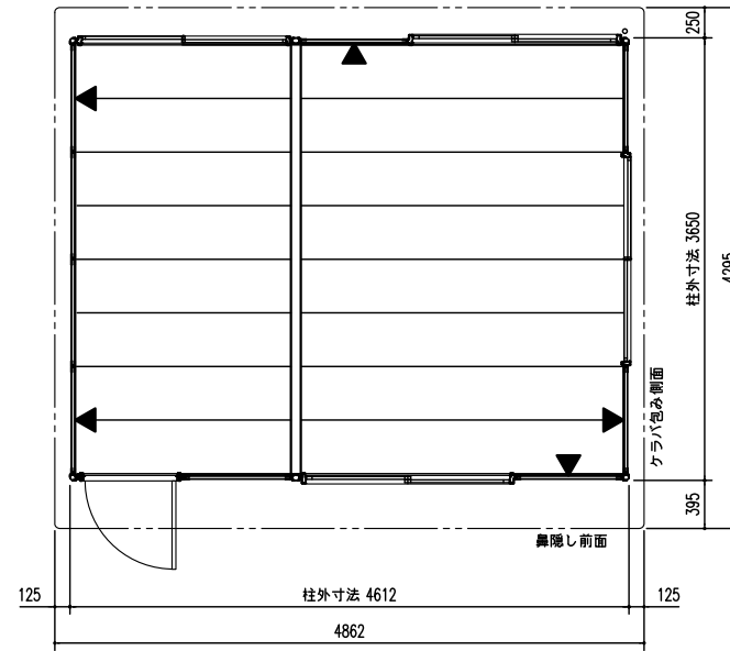
平面図 (S=1/50)
