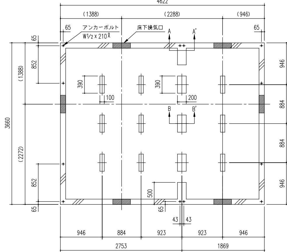
床 伏 図 (S=1/50)
