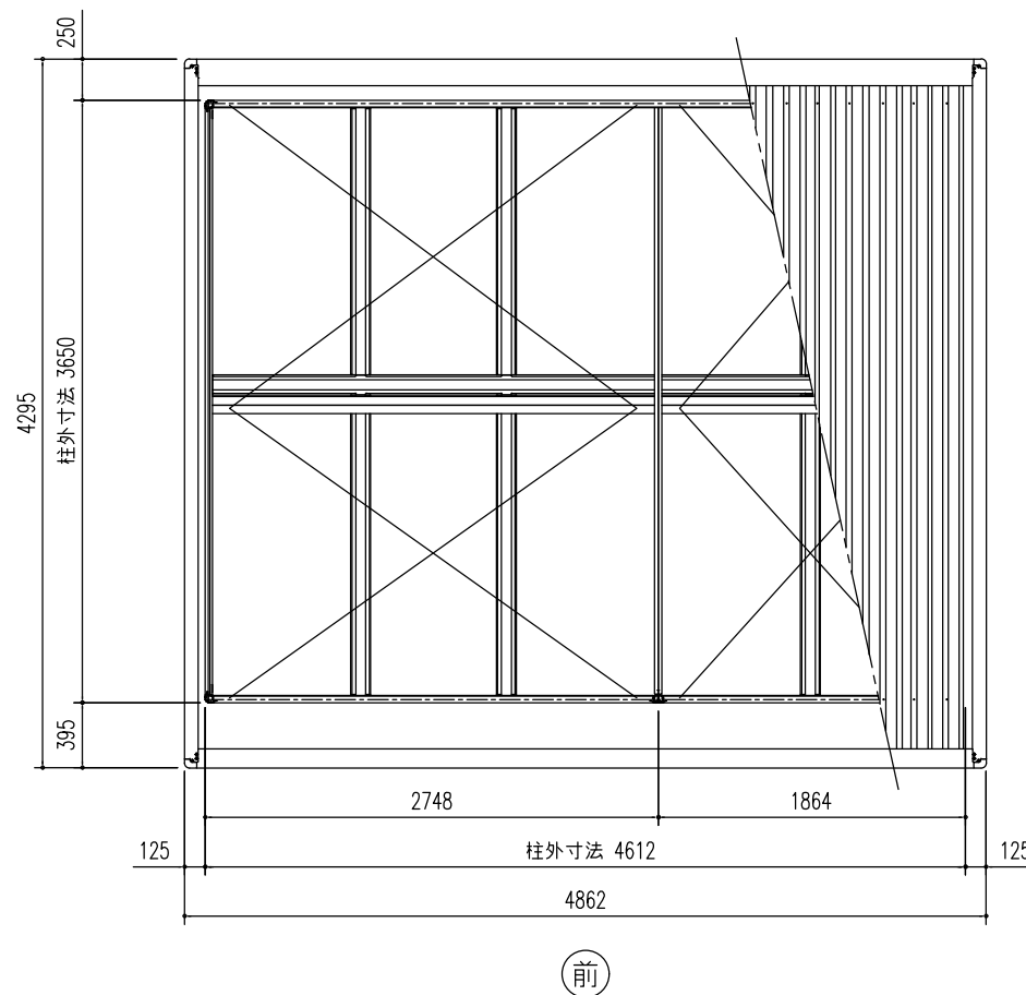
小 屋 伏 せ 図 (S=1/50)
