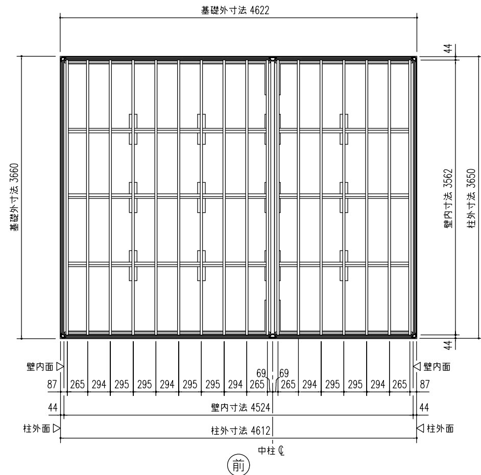
床 伏 図 (S=1/50)
