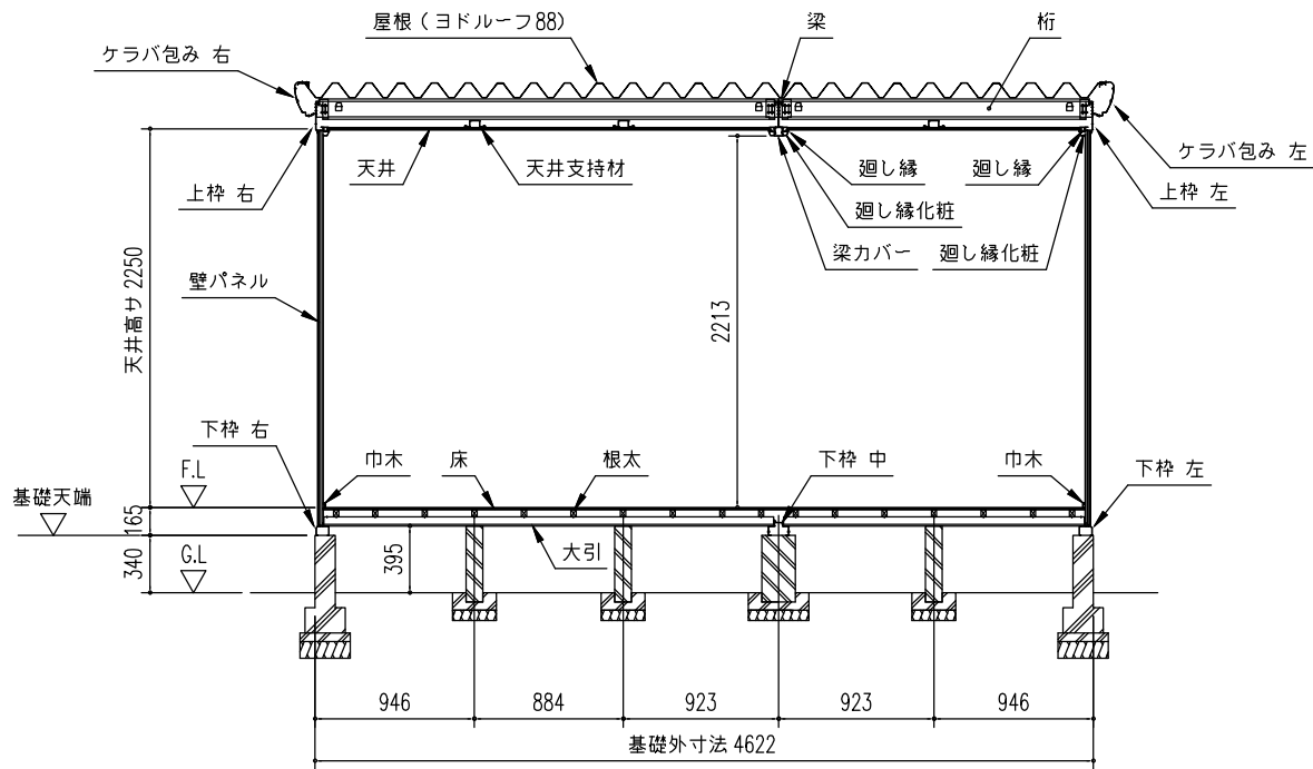
正面断面図 (S=1/50)
