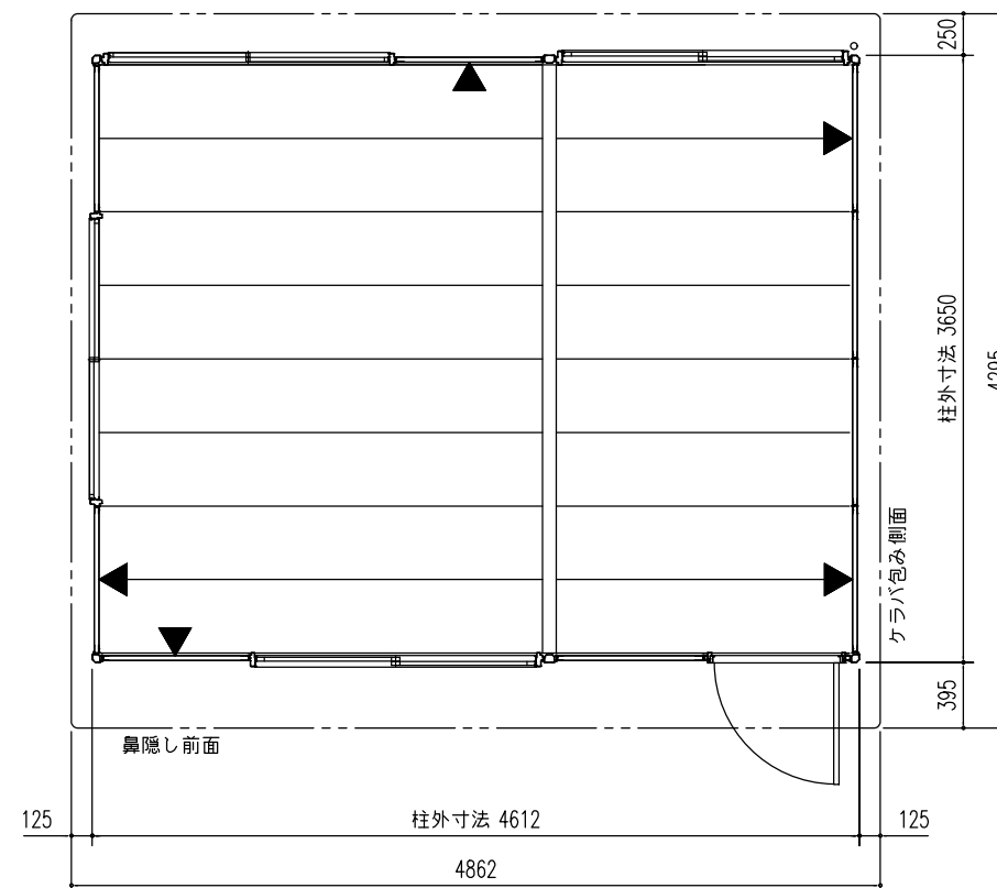
平面図 (S=1/50)
