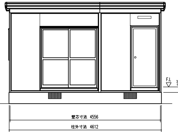
正面立面図 (S=1/50)
