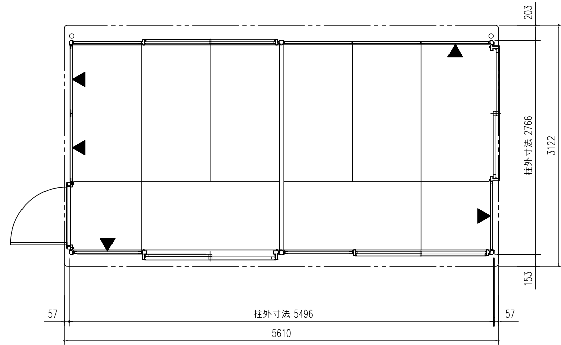
平面図 (S=1/50)
