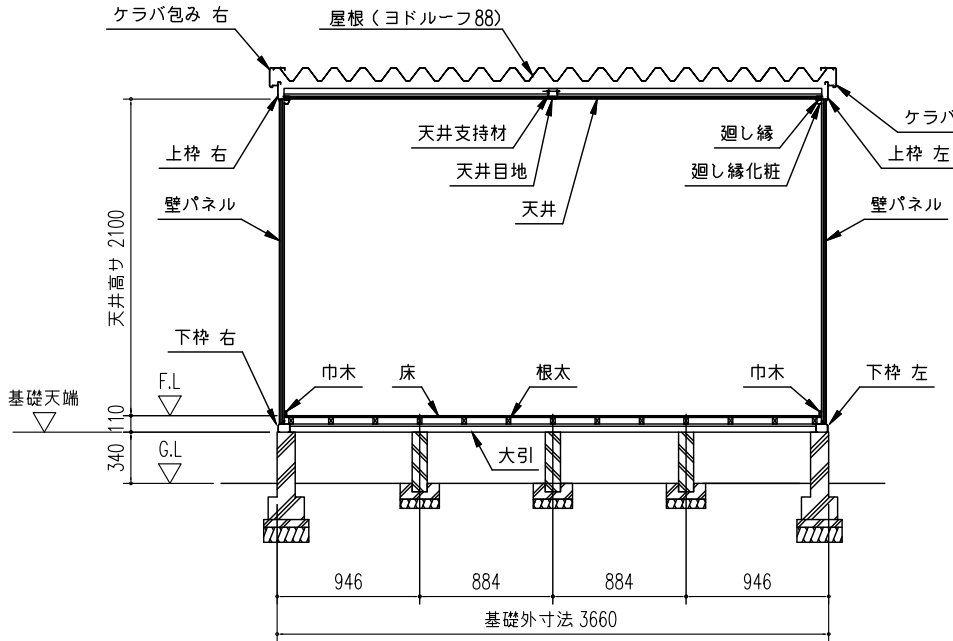
正面断面図 (S=1/50)
