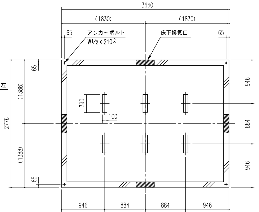
基礎図 (S=1/50)
