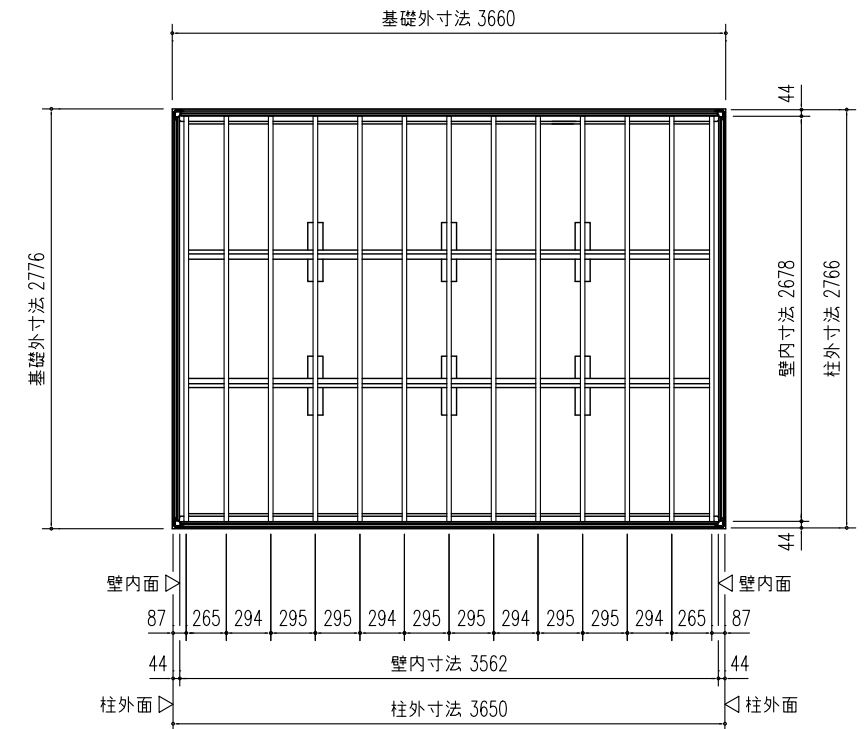
前 床伏図 (S=1/50)
