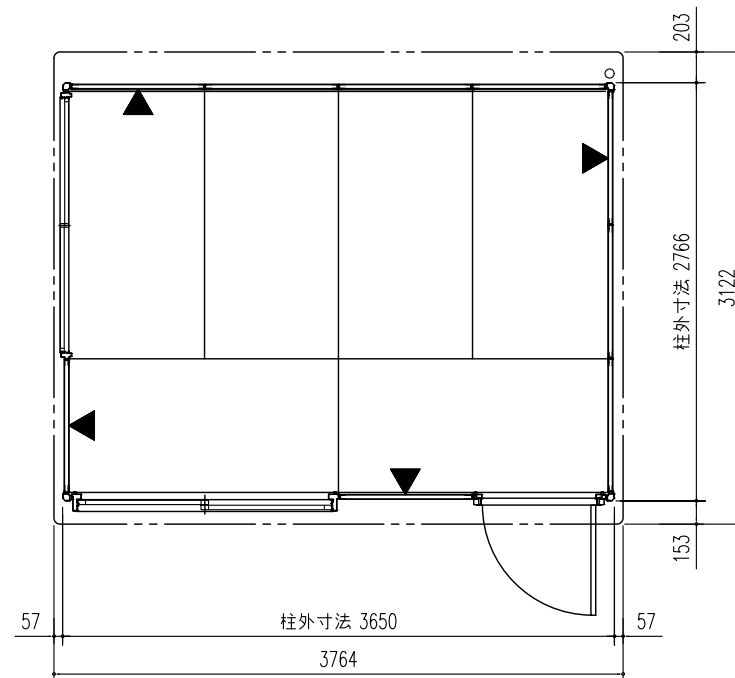
平面図 (S=1/50)
