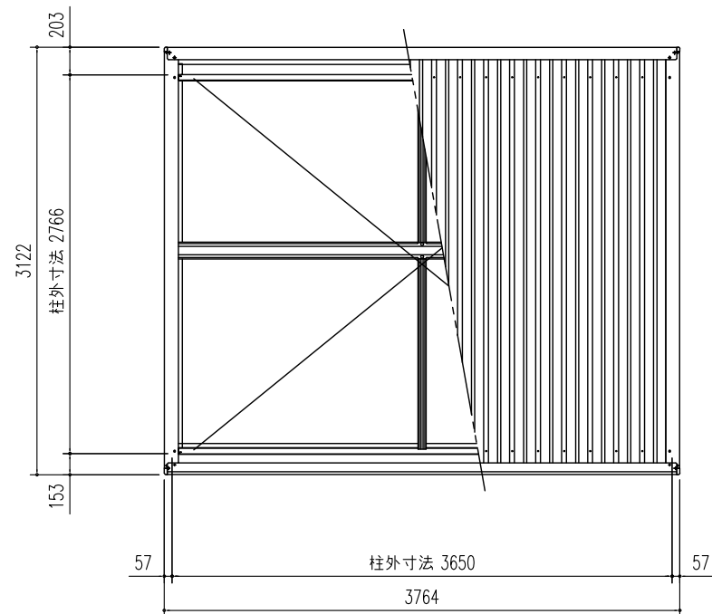
前 小屋伏せ図 (S=1/50)
