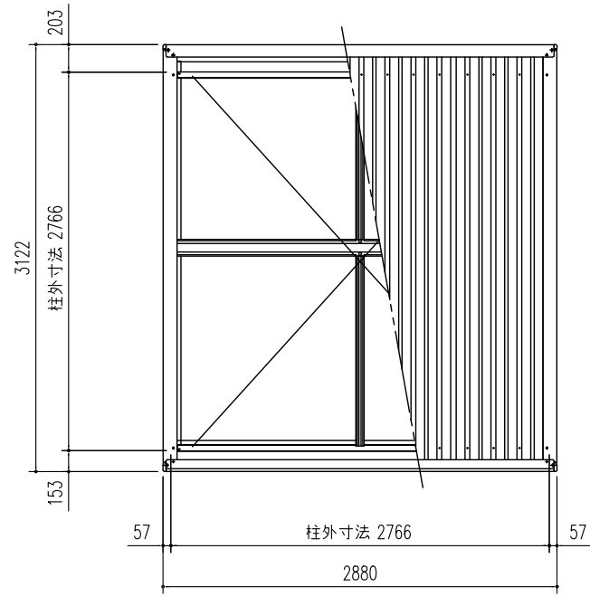
前 小屋伏せ図 (S=1/50)
