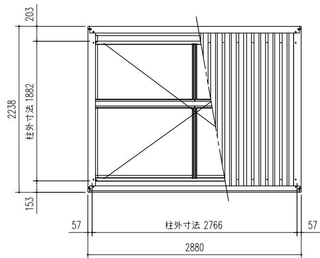
小屋伏せ図 (S=1/50)
