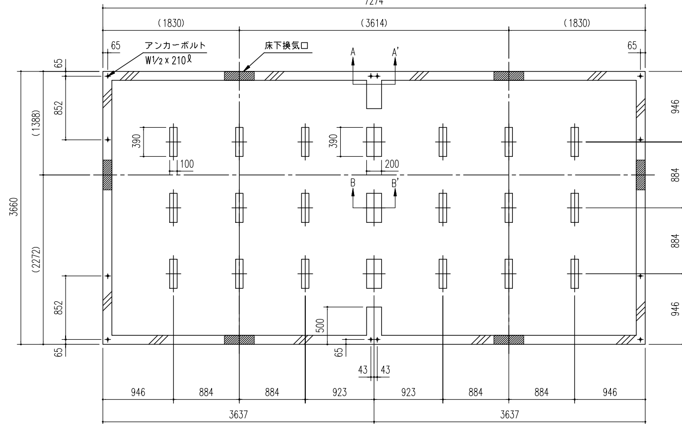
床 伏 図 (S=1/50)
