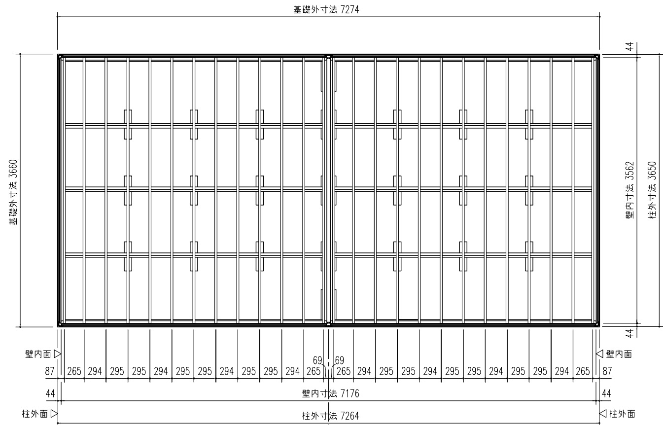
床 伏 図 (S=1/50)
