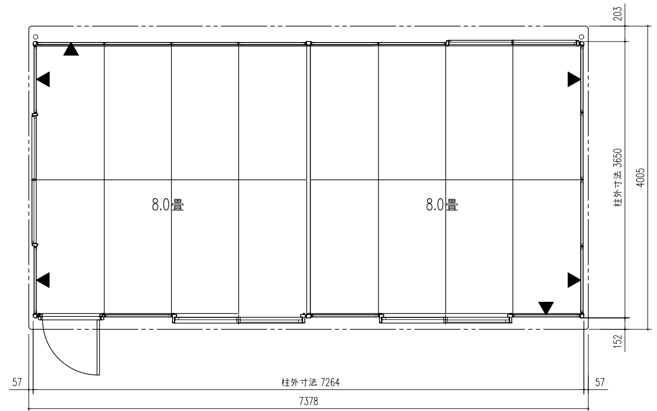
平面図 (S=1/50)
