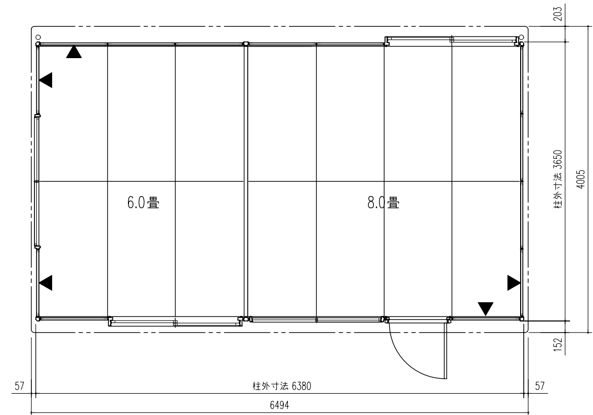
平面図 (S=1/50)
