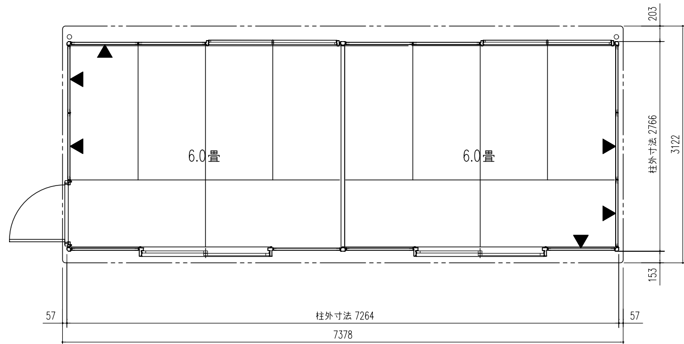
平面図 (S=1/50)
