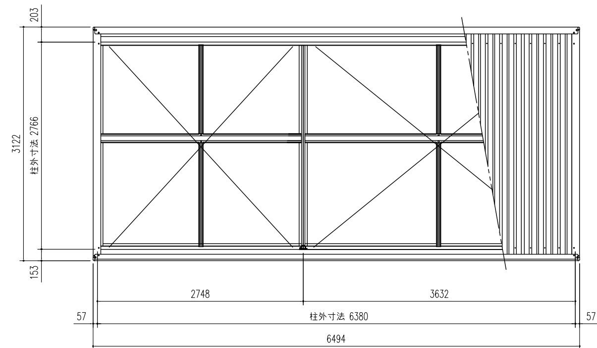
前 小 屋 伏 せ 図 (S=1/50)
