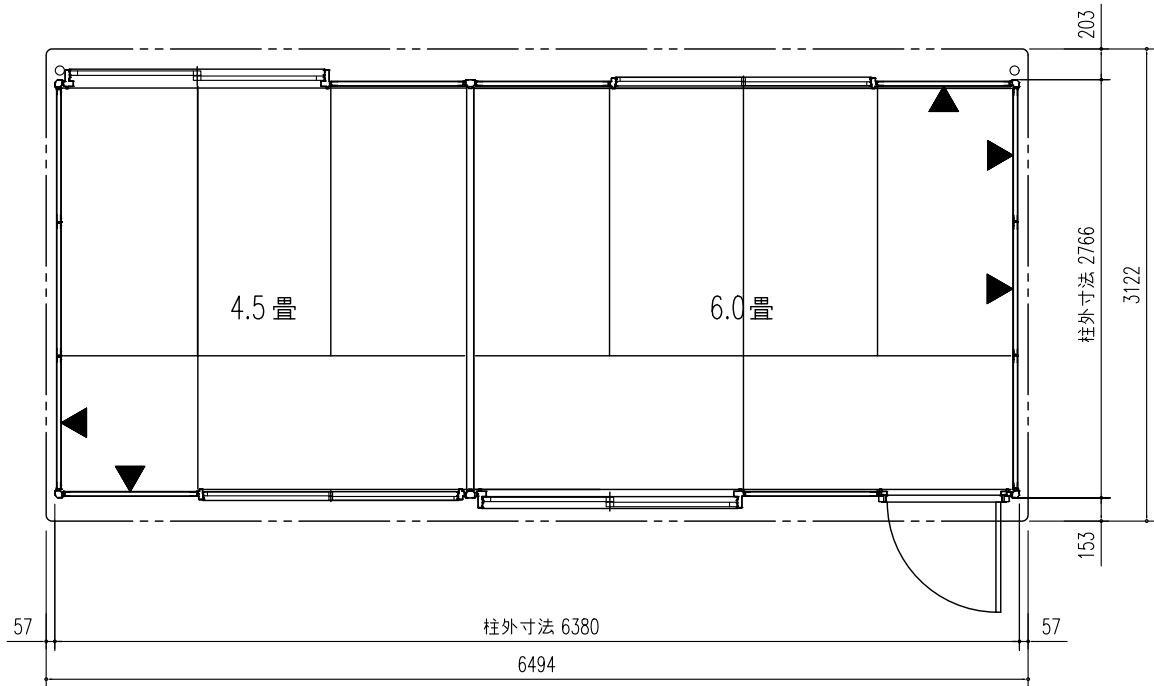
平面図 (S=1/50) ▼印はブレースパネルを示す。 間口 2枚 奥行 3枚
