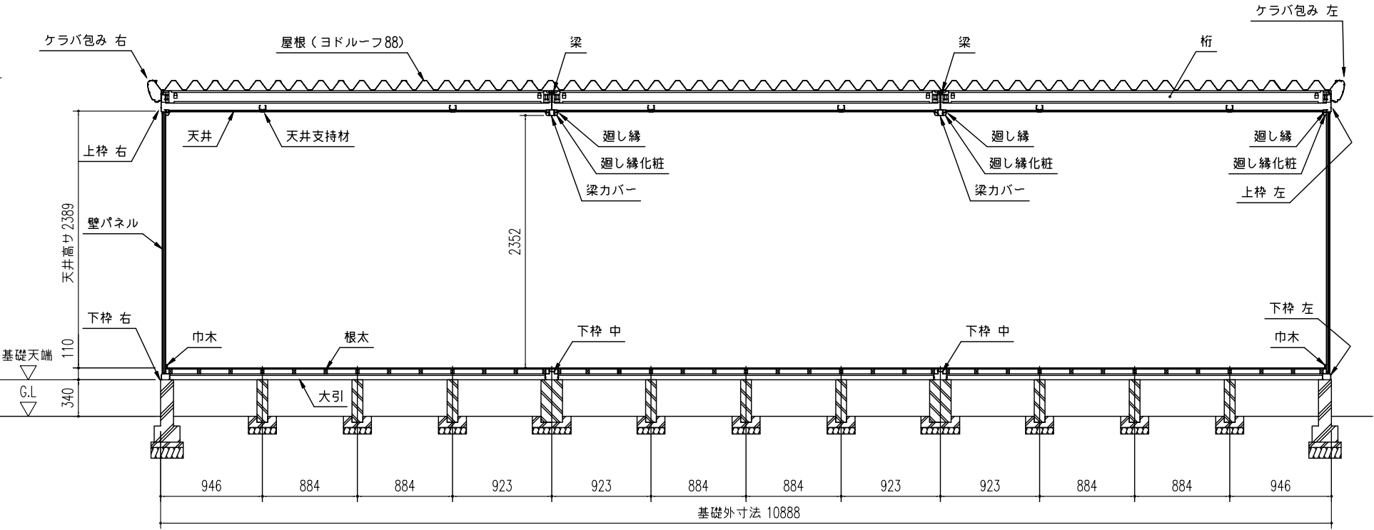
正面断面図 (S=1/50)
