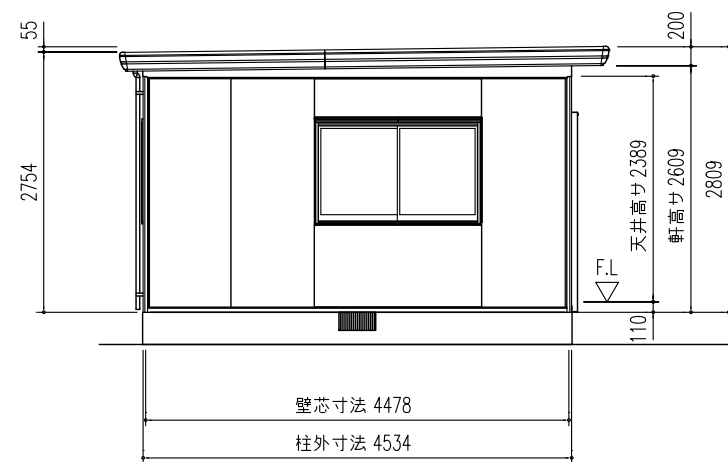
側面立面図 (S=1/80)
