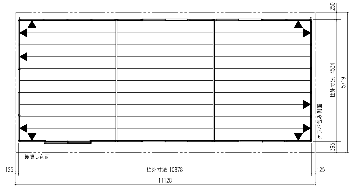
平面図 (S=1/80)
