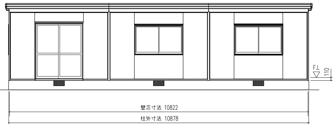
正面立面図 (S=1/80)
