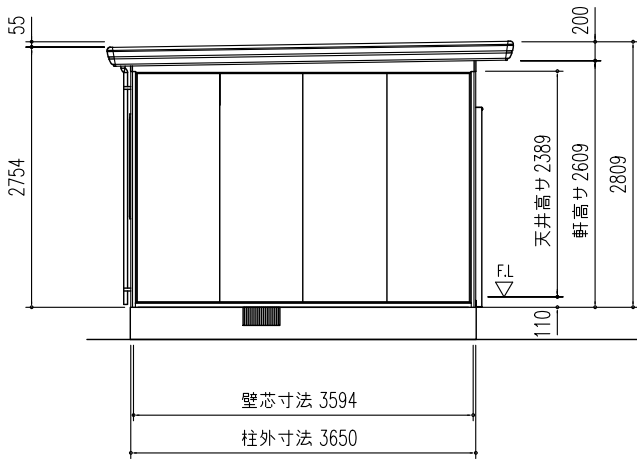
側面立面図 (S=1/80)
