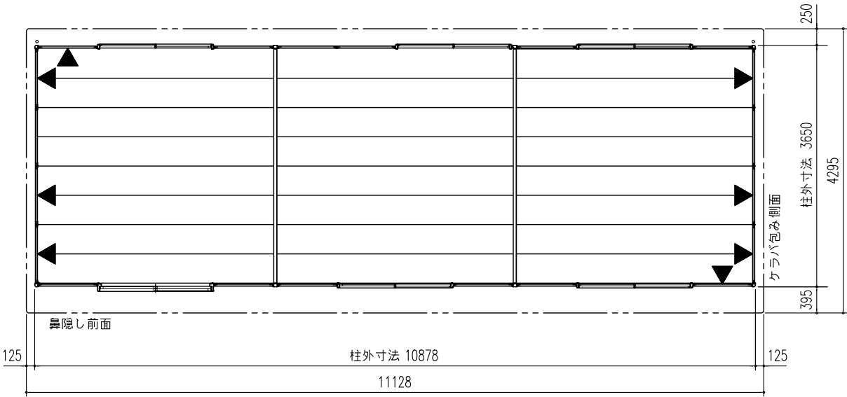
平面図 (S=1/80)
