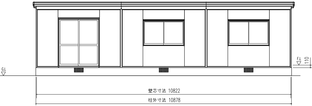
正面立面図 (S=1/80)
