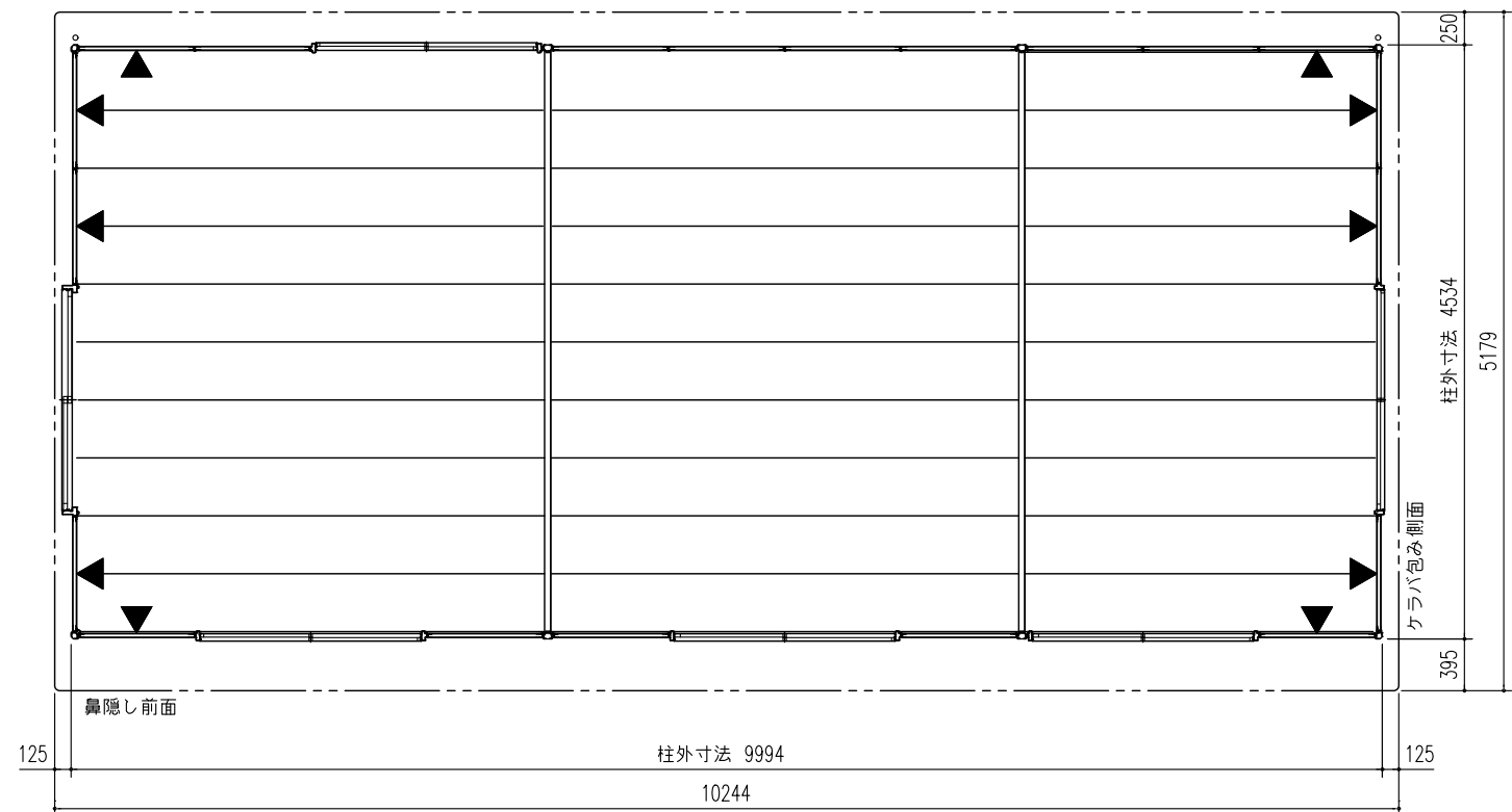
平面図 (S=1/60)
