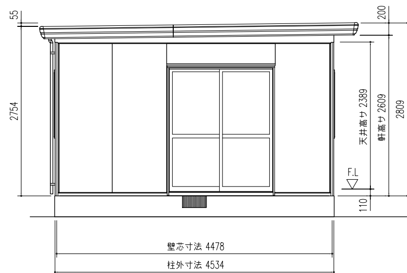
側面立面図 (S=1/60)
