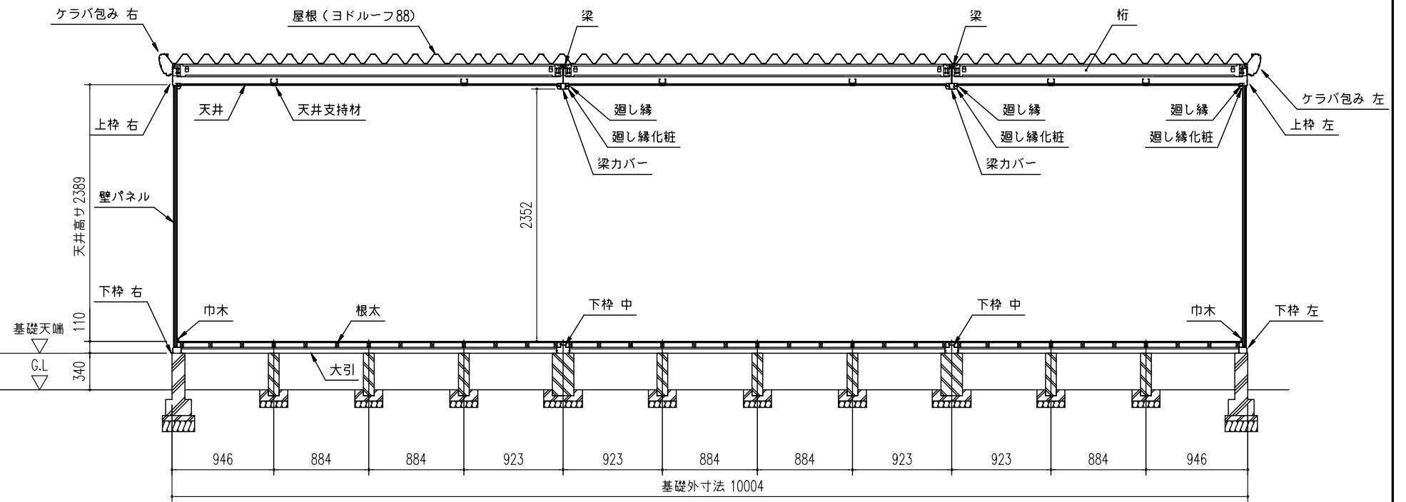
正面断面図 (S=1/50)
