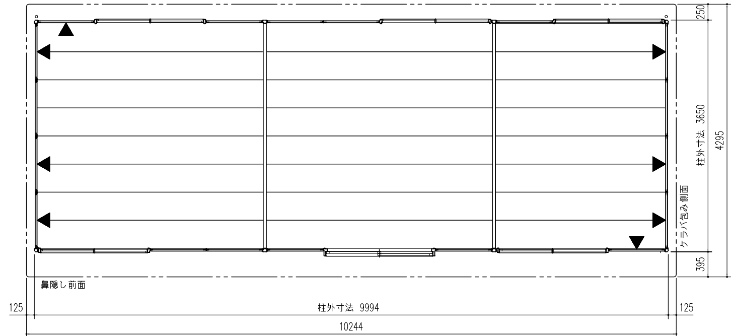
平面図 (S=1/60)
