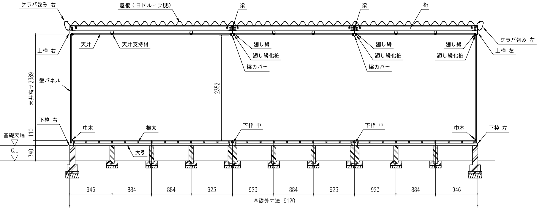
正面断面図 (S=1/50)
