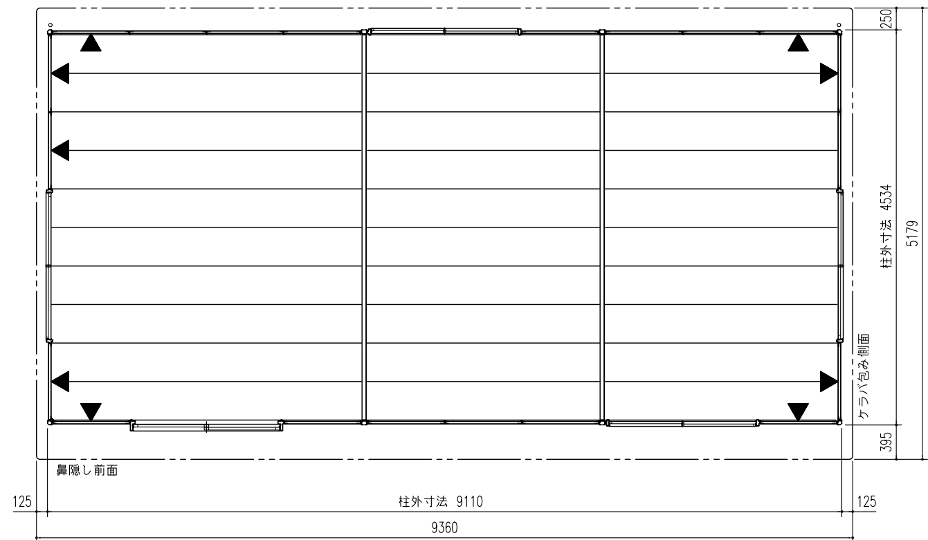
平面図 (S=1/60)
