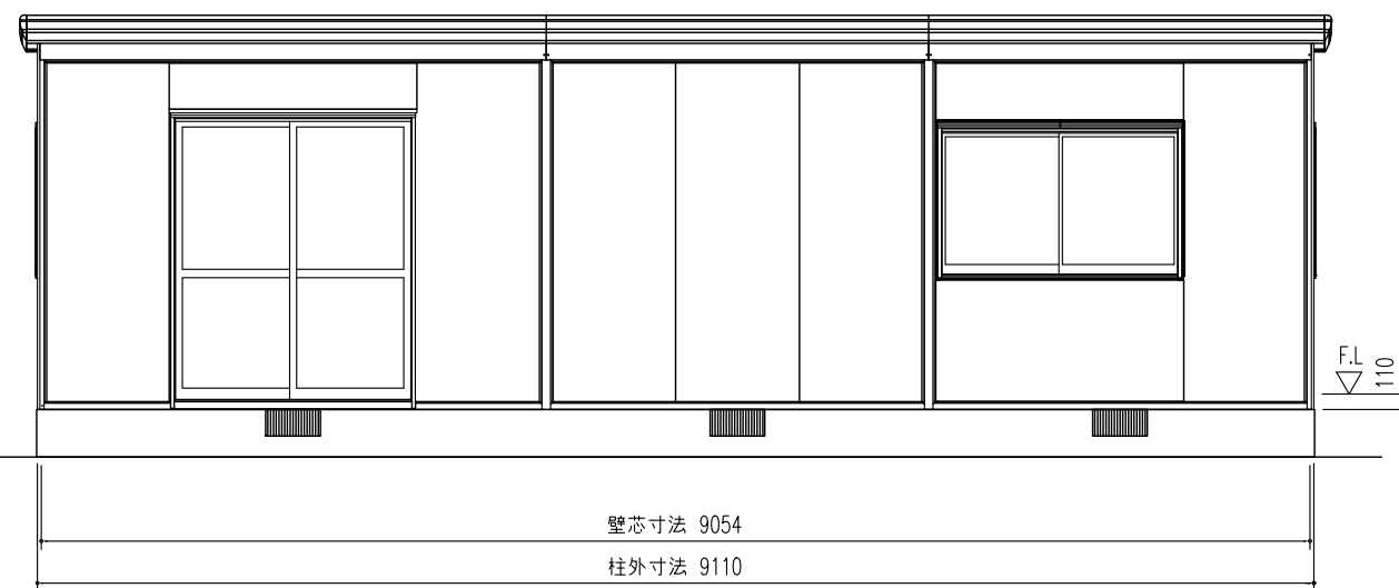
正面立面図 (S=1/60)
