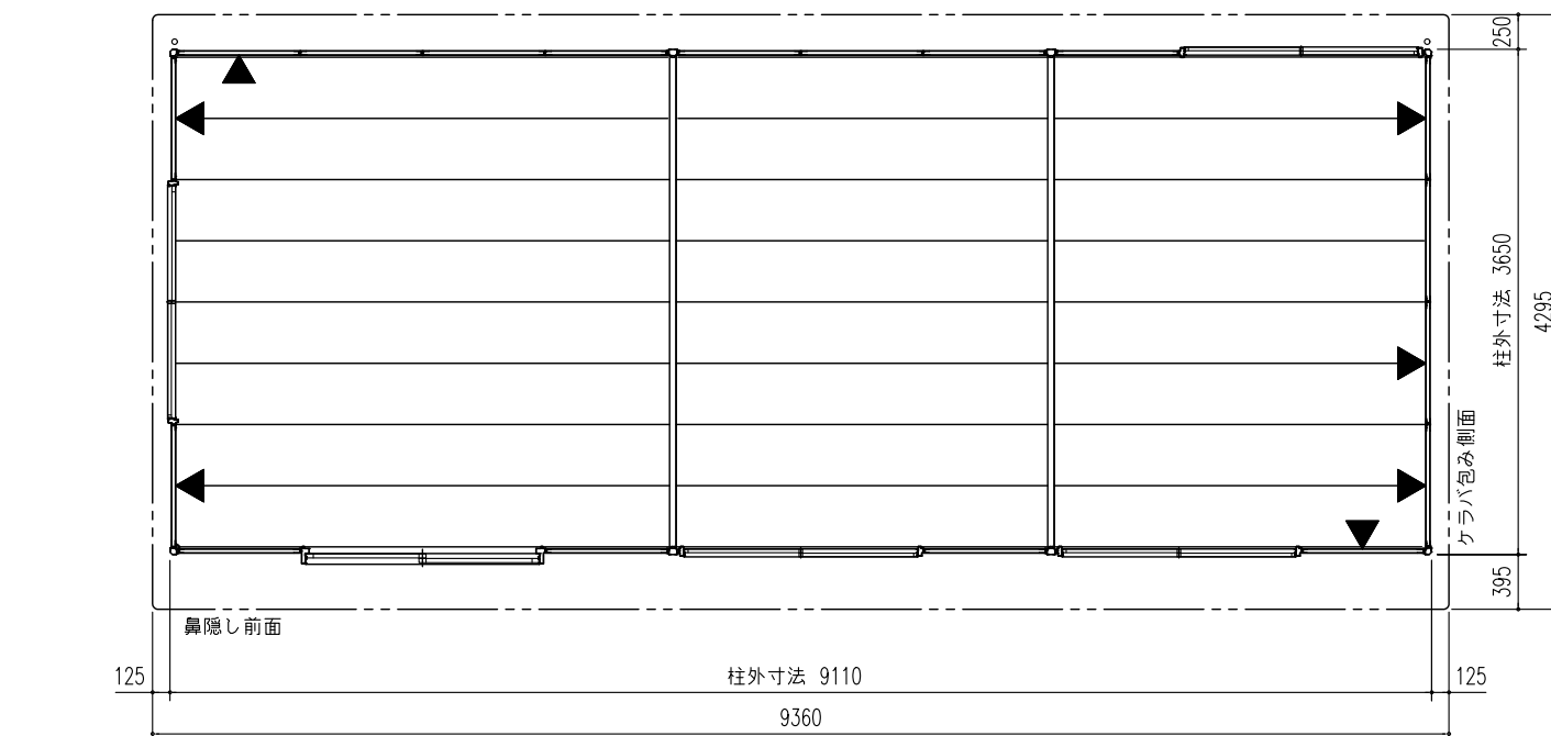
平面図 (S=1/60)
