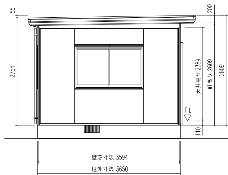
側面立面図 (S=1/60)
