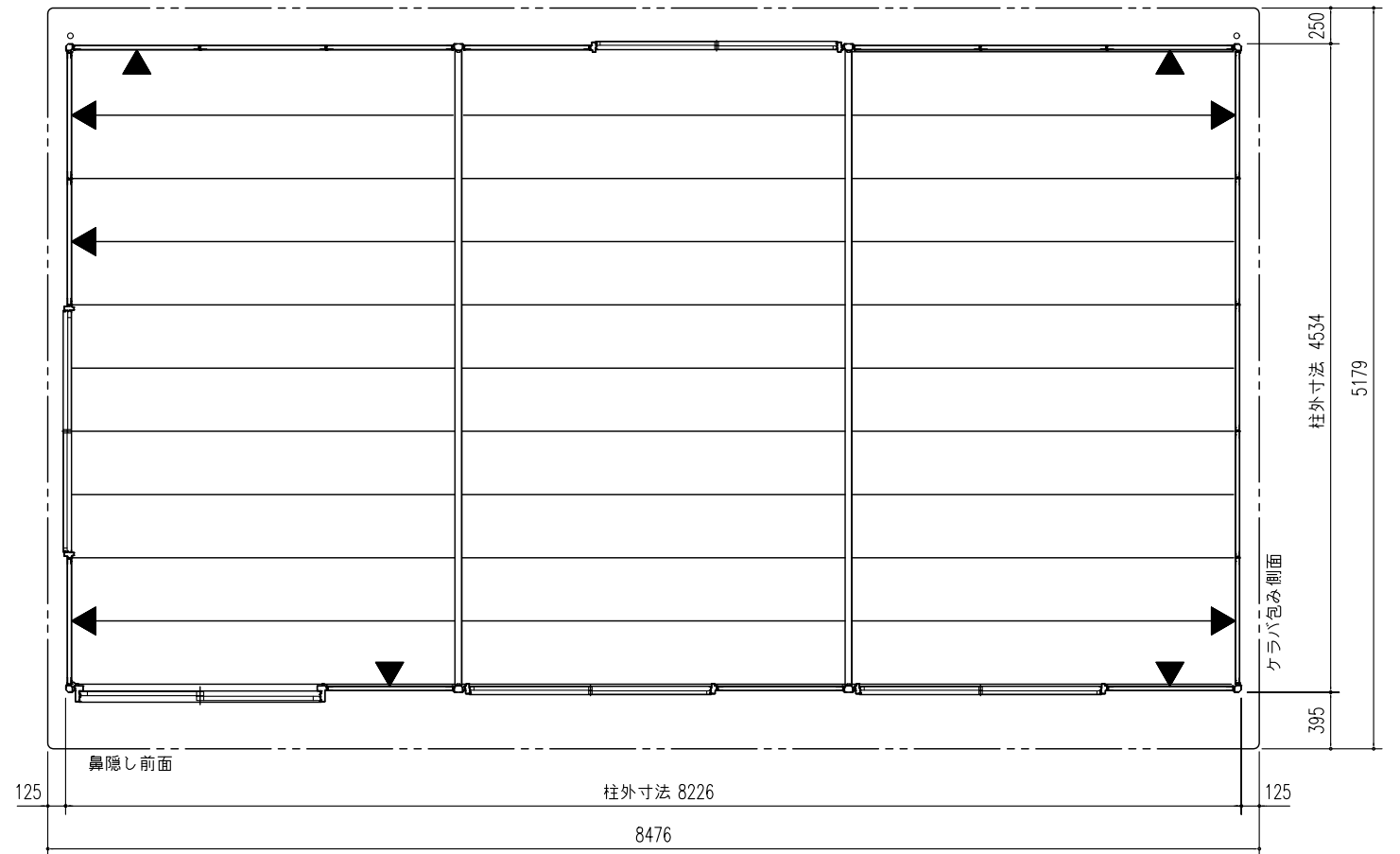
平面図 (S=1/50)
