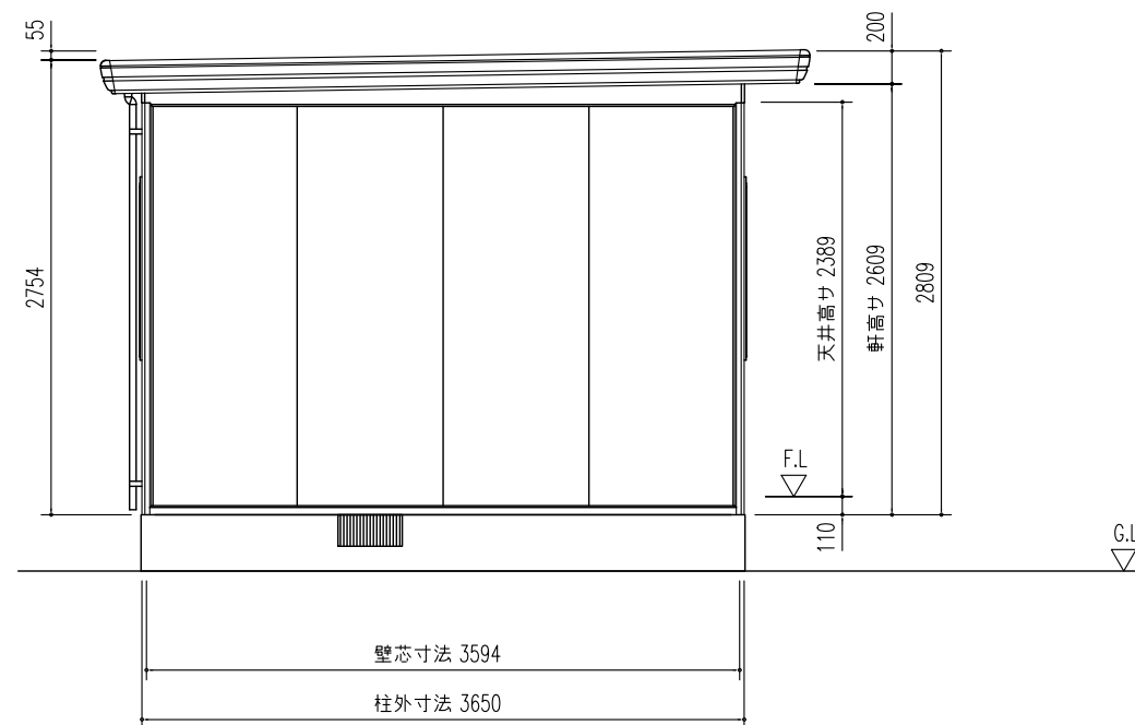
側面立面図 (S=1/50)
