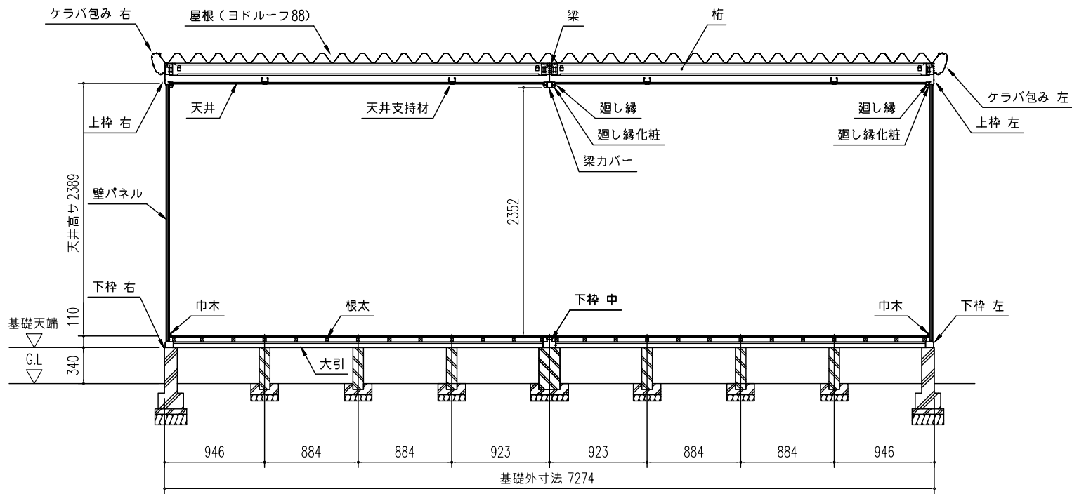
正面断面図 (S=1/50)
