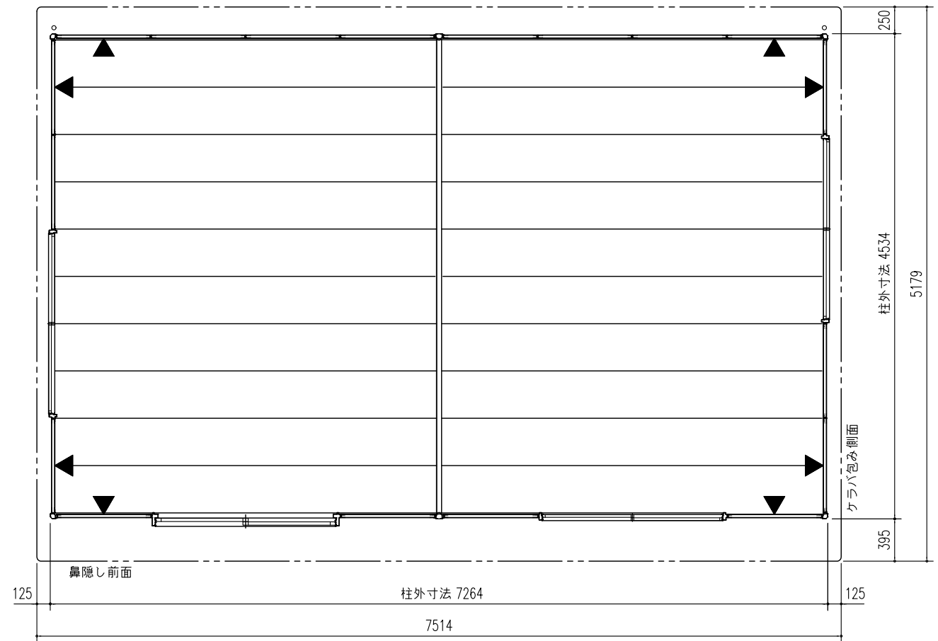
平面図 (S=1/50)
