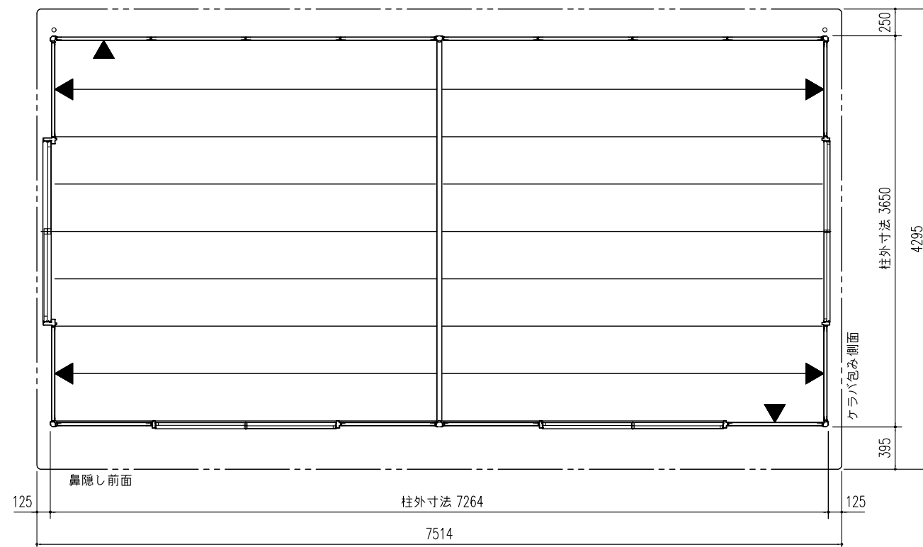
平面図 (S=1/50)
