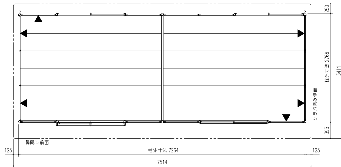
平面図 (S=1/50)
