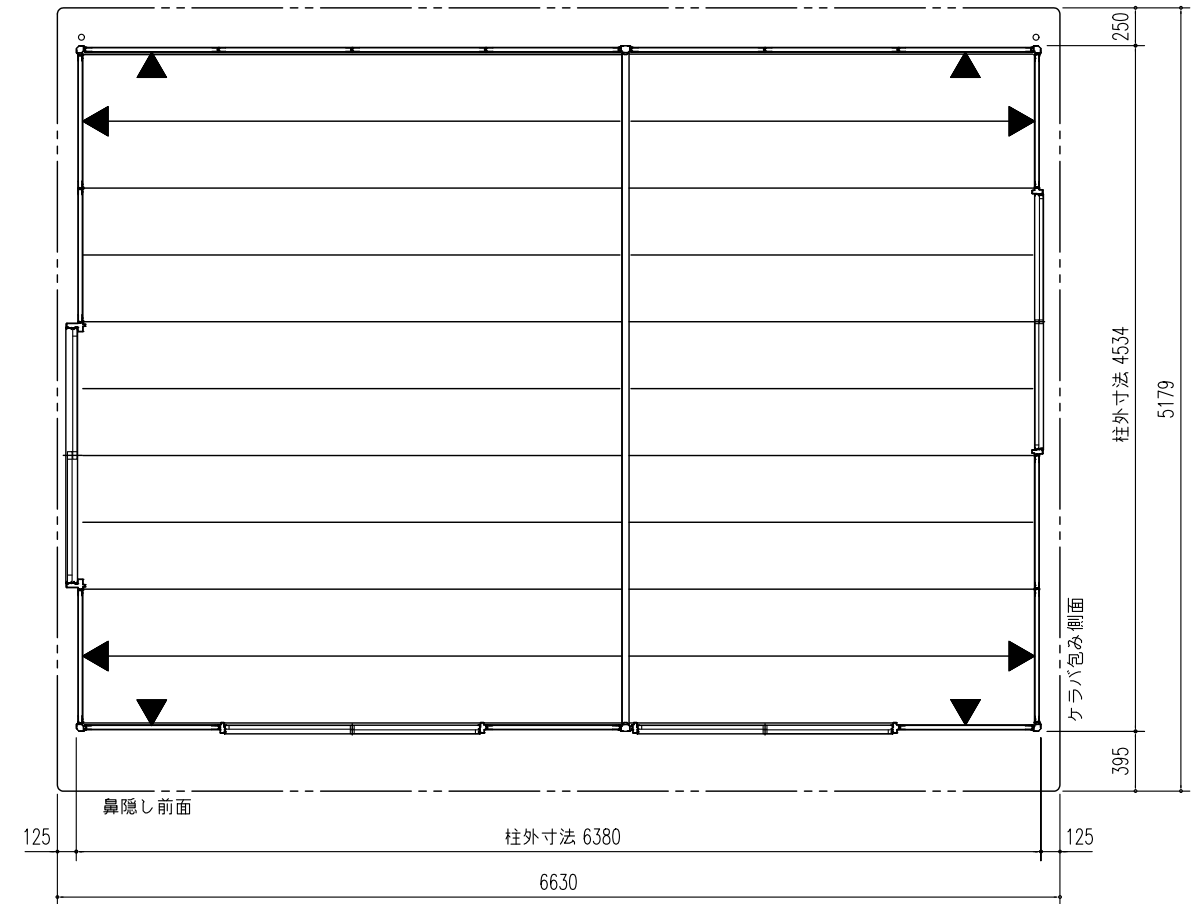
平面図 (S=1/50)
