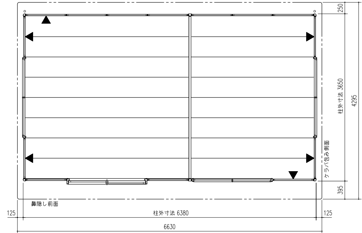
平面図 (S=1/50)
