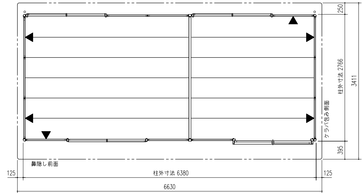
平面図 (S=1/50)
