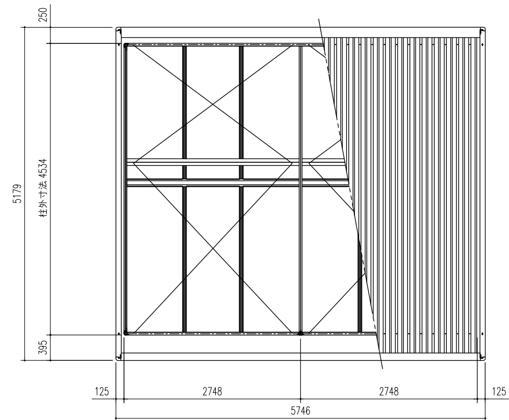
小 屋 伏 せ 図 (S=1/60)
