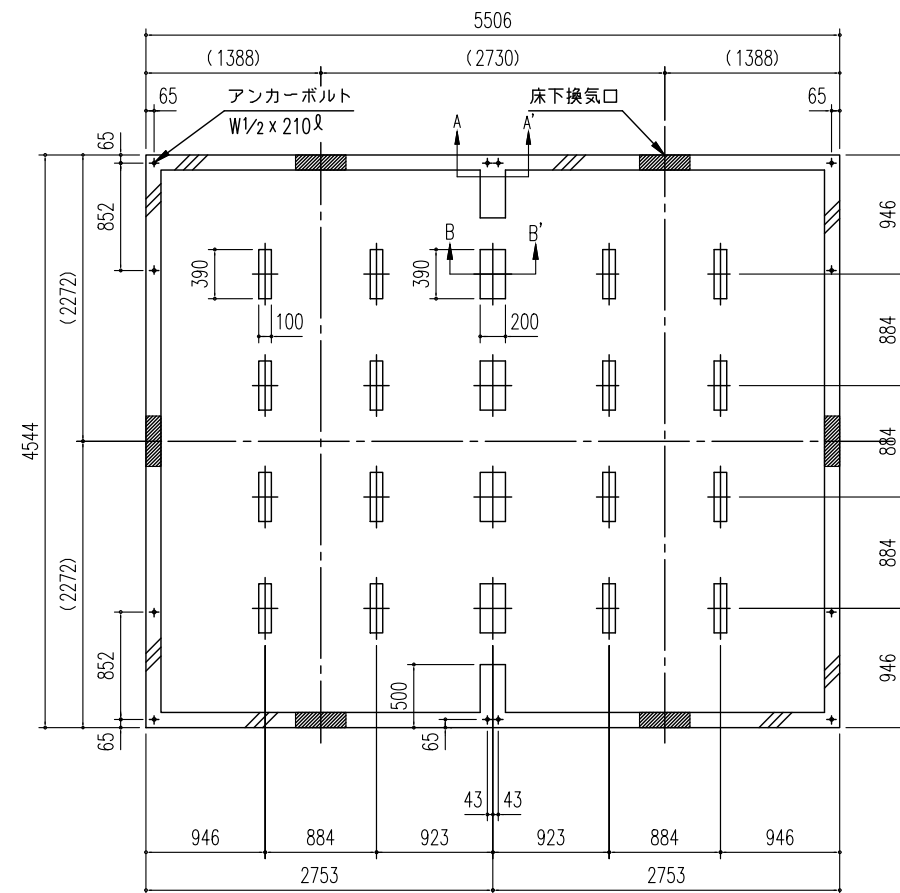
床 伏 図 (S=1/60)
