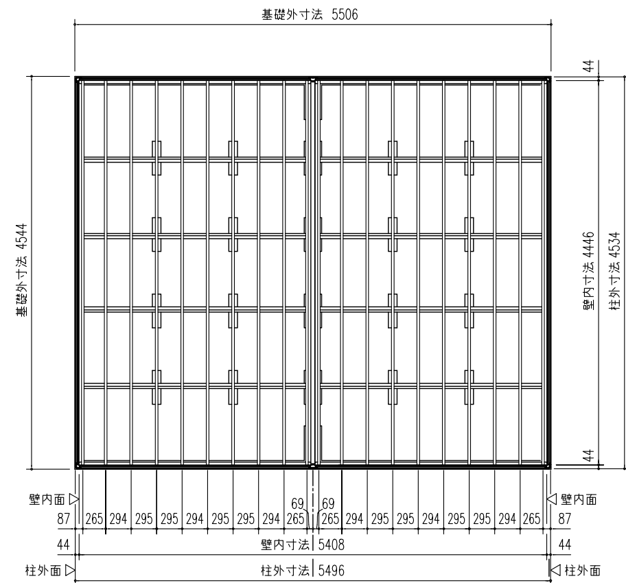
床 伏 図 (S=1/60)
