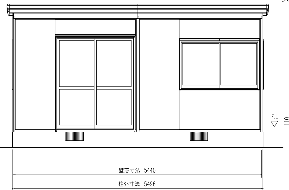
正面立面図 (S=1/50)
